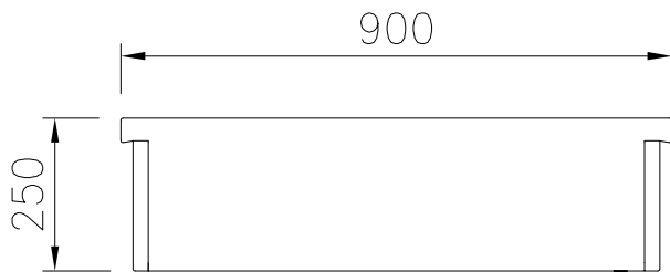
Zij aanzicht
